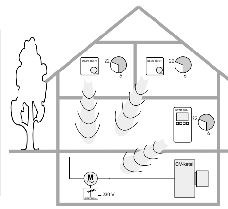
Afb 4: Pomplogica met master en slaves
