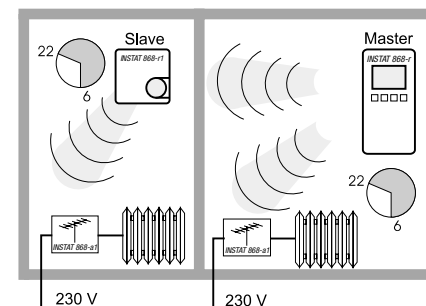
Afb 2: Enkelvoudige master/slave functie
